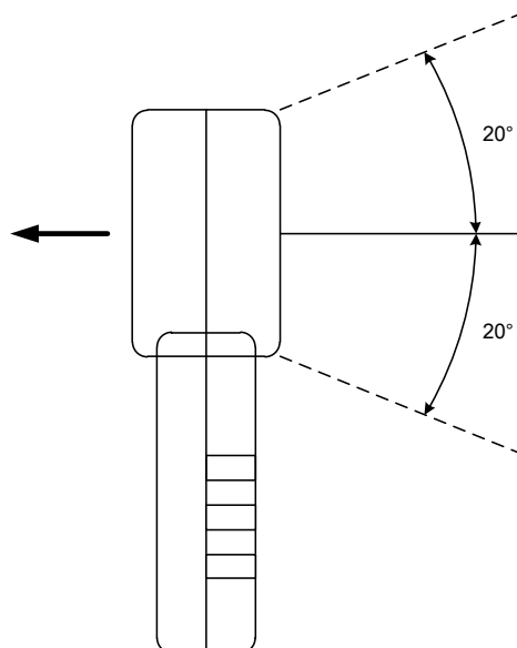
Figuur 2. Zorg dat de wind direct in de Anemometer blaast ( \pm 20 graden maximaal).
