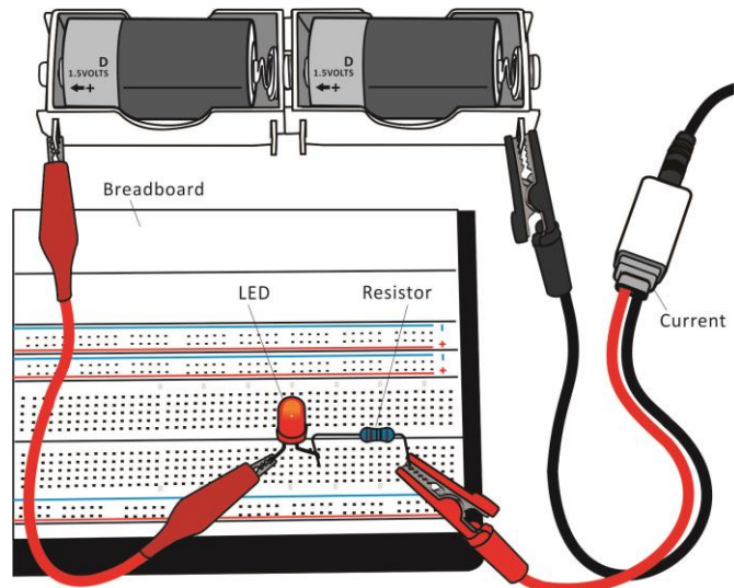
Figuur 2. Meten van de stroom die door een LED loopt.
